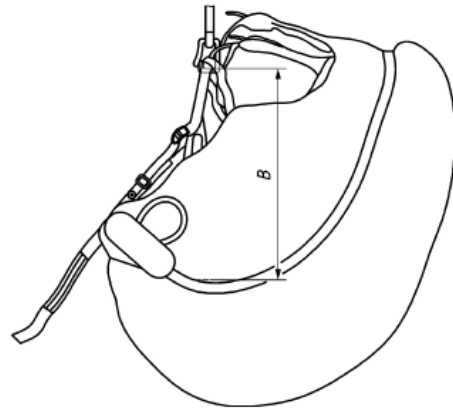
ハーネス取付位置の高さ Bild 6 — Höhe der Befestigungspunkte des Gurtzeugs
